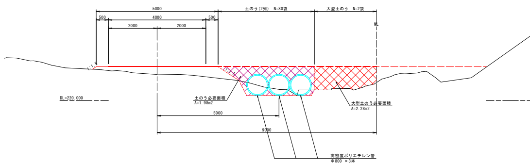
土のう構造図
