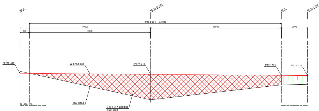
土留め土のう展開図 NO. 5~NO. 6付近 (R)
